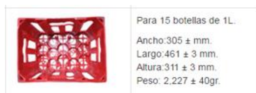
Figura 7. 2 Detalle de las cajas de Recogida Manual (Vidrio) 120 .
